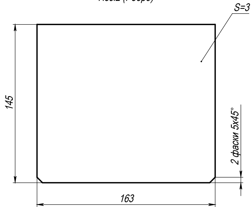
Поз.2 (Ребро)
